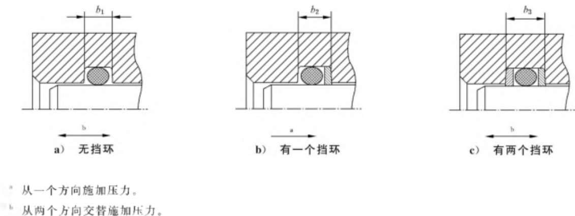
图 7 活塞杆密封挡环的安装位置
