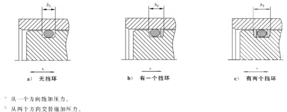
图 6 活塞密封挡环的安装位置
